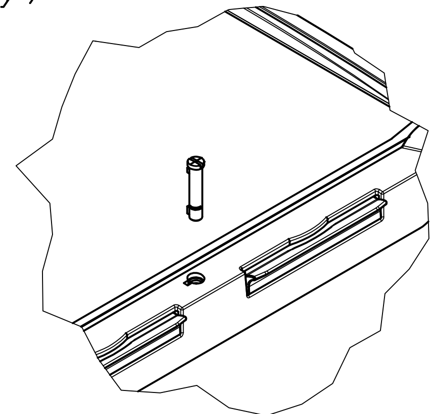
BCD-Sperrerr ( im Lieferumfang ) BCD catch ( included )
