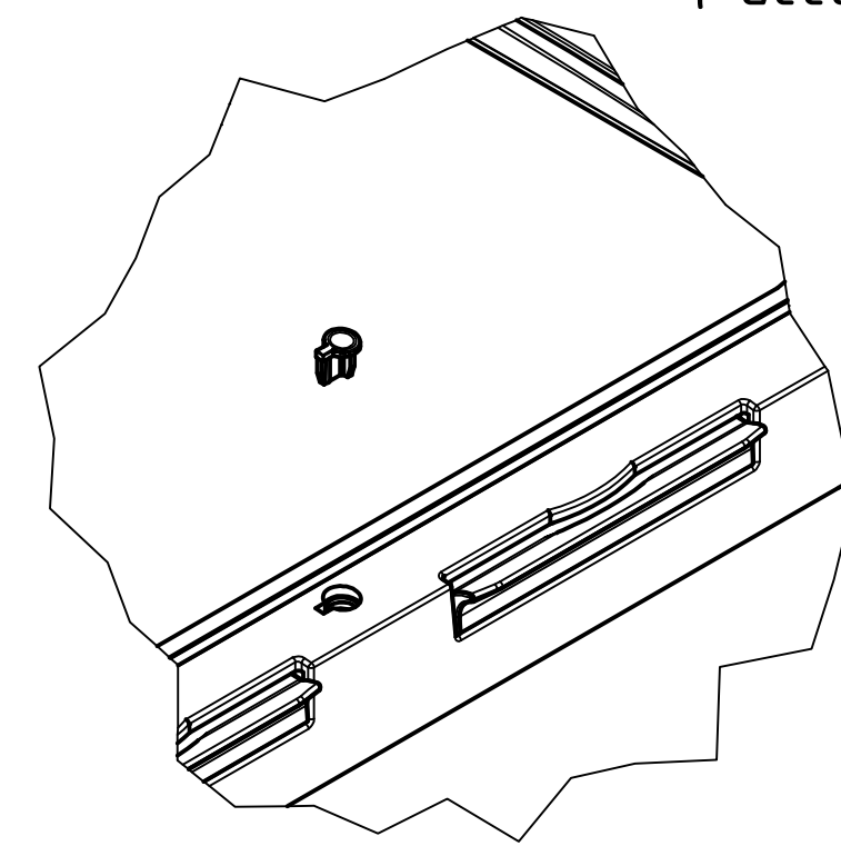
BCD-Schlossstopfen ( im Lieferumfang ) BCD blind plug ( included )
