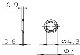
Sicherungsscheibe (BFS 0700)
